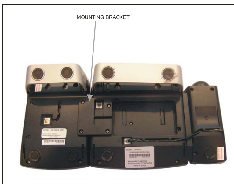
Figure 7.18 Attaching DS 64 Button Modules to a DS 5021D or a DS 5014D Keyset
